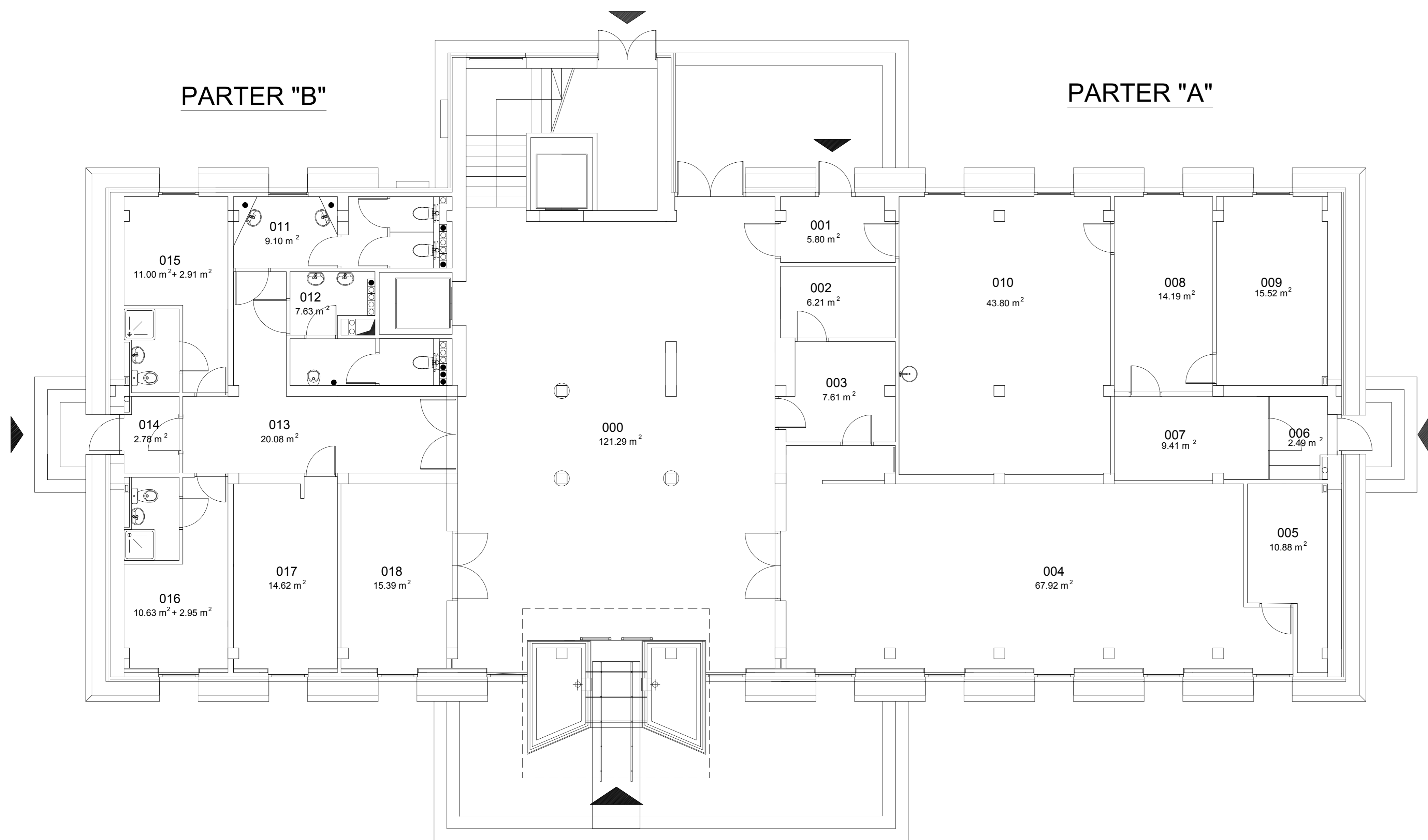
RZUT PARTERU
